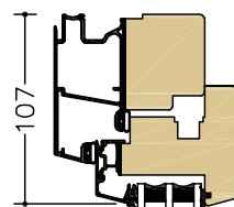
D-D Öppn./Fast Liggande karmpost
