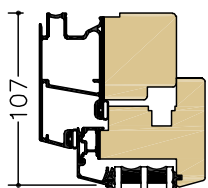
C-C Öppn./Öppn. Liggande karmpost
