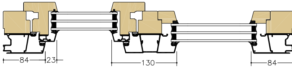
A-A TSD
