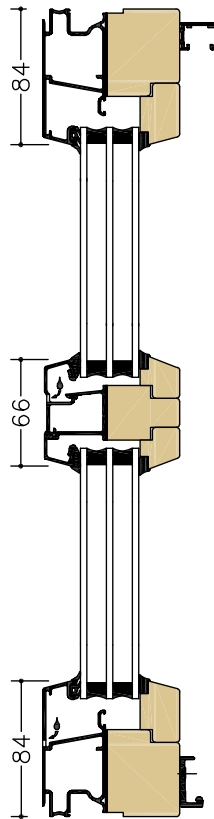
C-C TSD Fast del Karmpost
