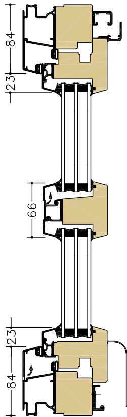
B-B TSD Skjutdel Bågpost
